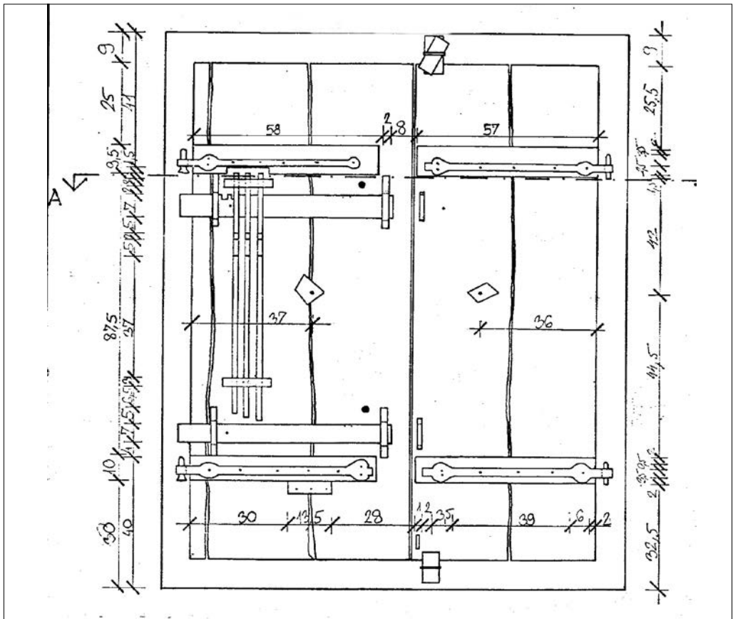
15. Pince bejáratú ajtó felmérése, belső oldal
