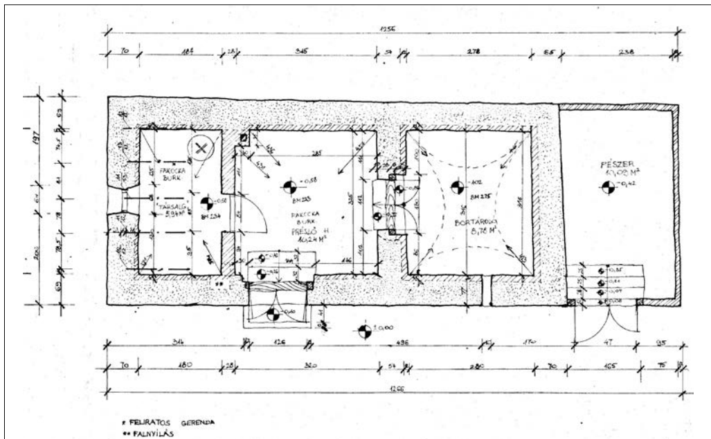
7. Pince alaprajz
