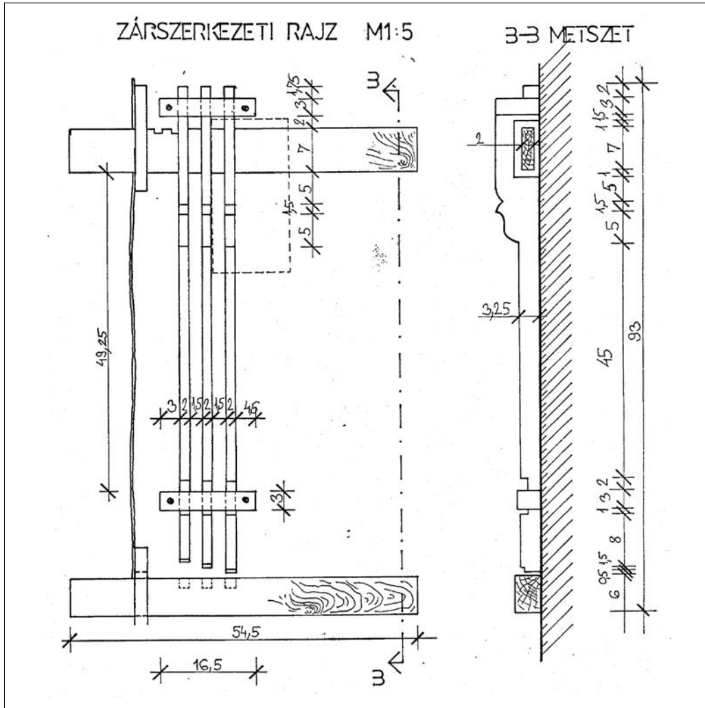
15. Pince bejáratú ajtó felmérése, belső oldal
