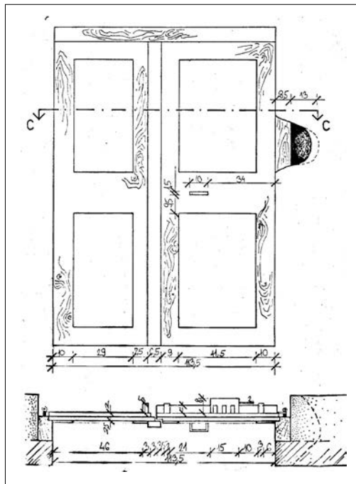
20. A bortároló ajtaja
