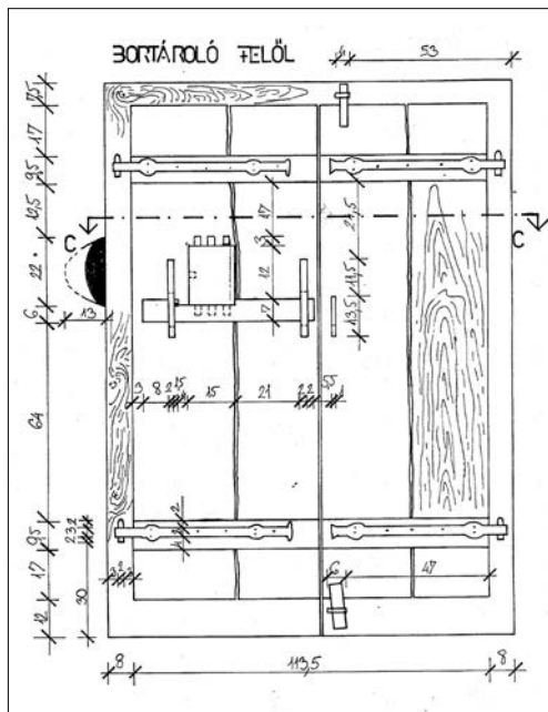
21. Fazárás ajtó belülről, a heveder elhúzva
