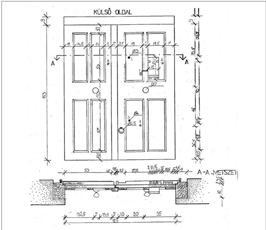
12. A pince bejárati ajtajának felmérése kívülről
